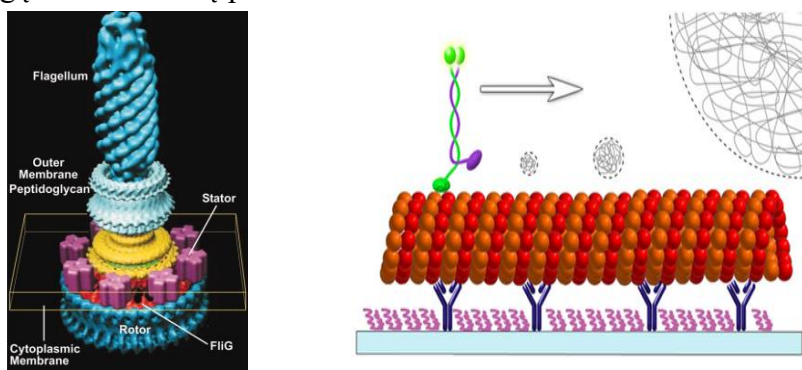
Ryc. 5.9. (a) "Wić" bakterii Escherichia coli jest prawdziwą nano-helisą, która obraca się dzięki zębatym wewnątrz komórki. (b) "Krok" kinezyne wzdłuż autostrady wewnątrz komórki wynosi około 8 nm, co 10 ms; kinezyne może przenosić bardzo duże obciążenia, jak samochód ciężarowy (K. SOZAŃSKI et al. ). ŹRÓDŁO: Wikipedia, American Physical Society.
