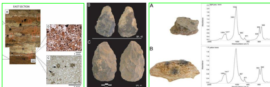
Ryc. 6.5. (a) Warstwa nr 10 z jaskini Wonderwerk zawierająca mikrogranulki popiołu. (b) Kamienne topory pochodzące z tej samej warstwy jaskini. c) Dwa fragmenty kości: powyżej fragment spalony w temperaturze 400^{\circ}\text{C} , poniżej nie-spalona kość; po prawej odpowiednie widma absorpcji w podczerwieni. ŹRÓDŁO: BERNA i in., „Proc. Natl. Acad. Sci. USA”, 2012.
