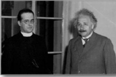
Ryc. 2.8. W 1933 po wykładzie Georges Lemaître'a w Princeton Einstein wykrzyknął: «To jest najpiękniejsze i najbardziej satysfakcjonujące wytłumaczenie stworzenia jakie kiedykolwiek słyszałem 13 ». Idea „początku czasu” została doceniona nawet przez Piusa XII w 1955 roku. ŹRÓDŁO: CATHOLIC EDUCATION RESOURCE CENTER, USA.
