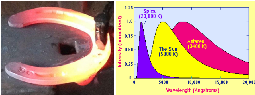
Ryc. 2.10. (a) Kolor podkowcy (i żarnika żarówki) zmienia się wraz z temperaturą: od czerwonego ( 1000^{\circ}\text{C} ), przez żółty, aż po biel światła żarówki w 3000^{\circ}\text{C} . (b) W taki sam sposób zmienia się kolor gwiazd: Spica z powierzchnią o temperaturze 23000^{\circ}\text{C} wydaje się błękitna w porównaniu ze Słońcem ( 5500^{\circ}\text{C} ), i z dużą, ale stosunkowo chłodną, czerwoną Antares (w Pasie Oriona). ŹRÓDŁO: NURE AGLIO; ERIC C. BLACKMAN (z podziękowaniami).
