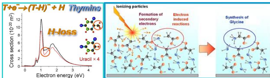
Ryc. 5.8. To elektrony o niskiej energii, powstające np. z promieniowania kosmicznego, niszczą wiązania między zasadami nukleotydowymi, umożliwiając "kołyszającym się" fragmentom tworzenie nowych mostów: mutacji (P. SCHEIER, Universität Innsbruck). (b) Te same powolne elektrony mogą (na określonej powierzchni, w warunkach wysokiej próżni i w niskiej temperaturze) wywoływać łączenie się \text{CH}_3\text{COOH} (kwasu octowego) z amoniakiem ( \text{NH}_3 ) w glicynę, najprostszy aminokwas. (A. LAFOSSE, Université Paris Sud).
