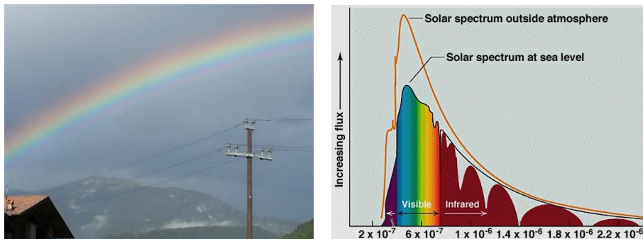
Rys. 2.9. (a) Tęcza w Villa Banale (Trydent); tęcza pojawia się, kiedy światło Słońca za nami, odbija się (i załamuje) w kroplach deszczu, które widzimy przed sobą. Pod siedmiokolorowym pasem widać również fukcję i magentę, które powstały w wyniku innego zjawiska optycznego: interferencji. Rozszczepienie białego światła na różne kolory jest przykładem „spektrum”, czyli widma. (b) Światło widzialne (tęcza) to tylko część spektrum Słońca, choć zawiera prawie 50% energii. Atmosfera tłumi nieco światło słoneczne, eliminując bardziej energetyczne światło ultrafioletowe. Ponadto dla podczerwieni atmosfera nie jest przezroczysta: zarówno H 2 O jak i CO 2 pochłaniają podczerwień.
