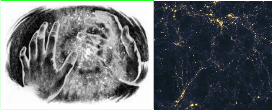
Ryc. 2.18. „Palec Boży” („Fingers of God”) strona z angielskiej Wikipedii z 2011 roku, dziś zmieniona. (b) Włókna galaktyk widziane w skali całego wszechświata: nie wiemy, dlaczego galaktyki łączą się w większe grupy zwane gromadami (mówi się o tajemniczej ciemnej materii jako o spoiwie), nie wiemy, dlaczego gromady tworzą włókna przypominające sieć, nie wiemy, czy Wszechświat rozszerza się poza jego widocznymi granicami. Nadal pozostaje więcej pytań niż odpowiedzi. ŹRÓDŁO: WIKIPEDIA 2011, 2019.
