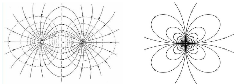
Ryc. 6.20. Wizualizacja pola elektrycznego (niewidocznego w naturze) wokół ładunków modelowych: (a) dwa przeciwstawne ładunki (dipol), (b) na zewnątrz cztery ładunki o tym samym znaku. Dzisiaj rozkład ładunków jest obliczany przez komputery, w latach 60-tych XX wieku, kiedy Feynman napisał swoje Wykłady z fizyki , trzeba było złożyć pewien rozkład, a następnie zweryfikować go punkt po punkcie. ŹRÓDŁO: R. FEYNMAN.
