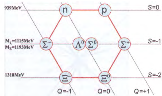
Rys. 2. Fenomenologiczne poszukiwanie struktury hadronów (czyli cząstek ciężkich ): oktet znanych w latach 60. barionów (czyli cząstek jądrowych ) o całkowitym spinie \frac{1}{2} , a będących kombinacją kwarków u, d i s: na osi pionowej „dziwność” (czyli liczba kwarków strange ), po skosie – ładunek elektryczny. W środku znajduje się (nietrawny) hiperon \Lambda , który może zastąpić neutron w jądrze atomowym
