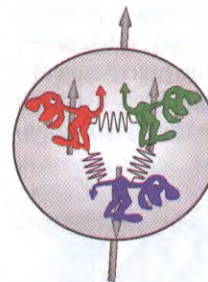
Rys. 3. Użyjmy wyobraźni: kwarki nie jako kropczki. Proton składa się z dwóch kwarków up i jednego down . Całkowity spin protonu wynosi \frac{1}{2} . Idea: G.K., rysunki: dr T. Wróblewski, © 2003 [1]
