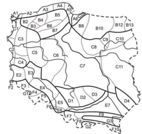
Rys. 16.4. Regionalizacja klimatu Polski E. Romera
