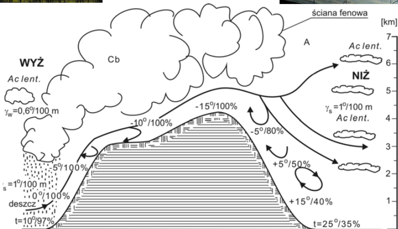
Rys. 9.15. Schemat powstawania wiatru fenowego (halnego)
