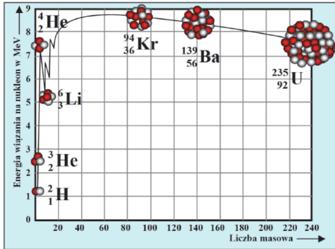
Ryc. 3.10. a) Produkty rozszczepienia uranu ^{235}\text{U} (na dwa fragmenty) obejmują szeroki rozkład izotopów od A = 70 do A = 170 ; zwróć uwagę, że skala pionowa jest względna (0,1, 1, 10); b) energia wiązania na jeden nukleon w zależności od liczby masowej A ; cząstka alfa, czyli ^4\text{He} ma dużą energię wiązania; maksimum krzywa osiąga około żelaza ^{56}\text{Fe} ; dla jąder poniżej masy żelaza korzystna energetycznie jest synteza, powyżej żelaza – rozszczepienie (Źródło: European Nuclear Society)
