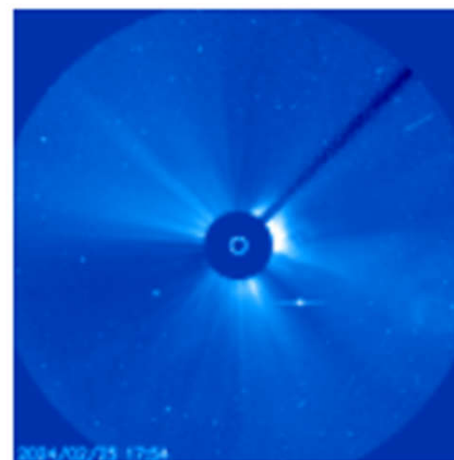
LASCO C3
