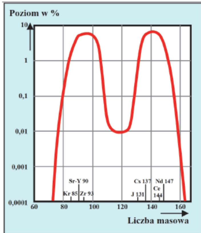
Ryc. 3.10. a) Produkty rozszczepienia uranu ^{235}\text{U} (na dwa fragmenty) obejmują szeroki rozkład izotopów od A = 70 do A = 170 ; zwróć uwagę, że skala pionowa jest względna (0,1, 1, 10); b) energia wiązania na jeden nukleon w zależności od liczby masowej A ; cząstka alfa, czyli ^4\text{He} ma dużą energię wiązania; maksimum krzywa osiąga około żelaza ^{56}\text{Fe} ; dla jąder poniżej masy żelaza korzystna energetycznie jest synteza, powyżej żelaza – rozszczepienie (Źródło: European Nuclear Society)
