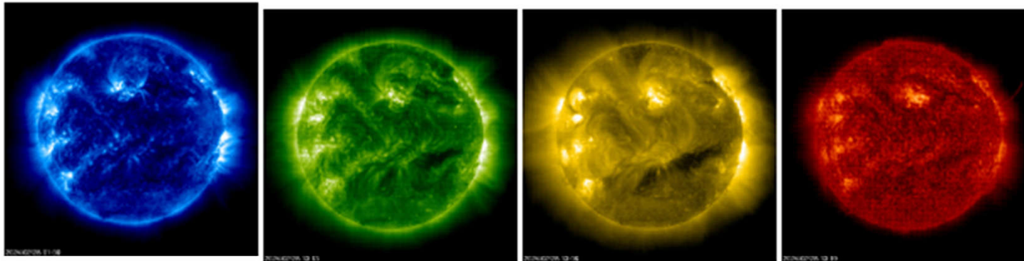
EIT 171 (1.000.000 K)
