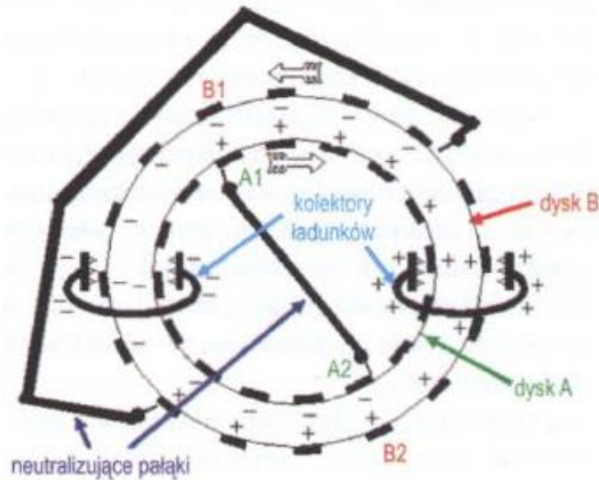
Rys. 2. Schemat rozmieszczenia ładunków w maszynie elektrostatycznej Wimshurst'a [4]. Jeżeli na jednej z pinezek, A1, powstanie ładunek dodatni, to przez indukcję na pinezce B1 naprzeciw (tj. na drugim dysku), powstanie ładunek ujemny
