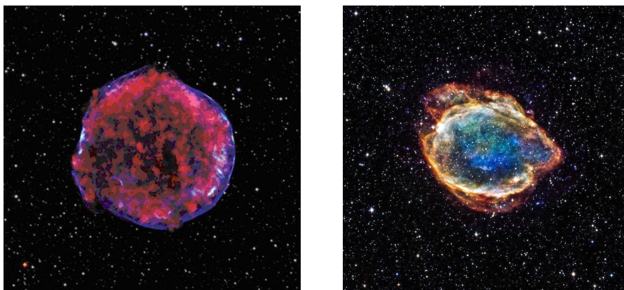
Ryc. 2.16. (a) Pozostałości supernowej AD 1572 (Tycho Brahe) w promieniowaniu rentgenowskim: na czerwono promienie o małej energii, na niebiesko promienie o dużej energii. (b) Pozostałości supernowej (G299), prawdopodobnie widocznej gołym okiem 4500 lat temu. ŹRÓDŁO: CHANDRA.HARVARD.EDU.
