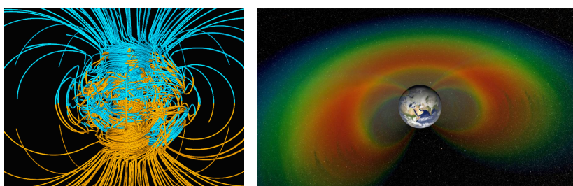
Rysunek 4.9. (a) Model dynamo magnetycznego Ziemi: skomplikowana struktura pola na powierzchni Ziemi jest spowodowana „skłębieniem się” linii wewnątrz żelaznego jądra, gorącego i kręcącego się (razem z całym globem). (b) Pole magnetyczne zabezpiecza nas przed napływem energetycznych cząstek ze Słońca (wiatrem słonecznym), które są niebezpieczne dla życia. Cząstki te zostają zogniskowane przez pole magnetyczne nad biegunami: obserwujemy zorzę polarną. ŹRÓDŁO: GARY A. GLATZMAIER; NASA/Goddard Space Flight Center.
