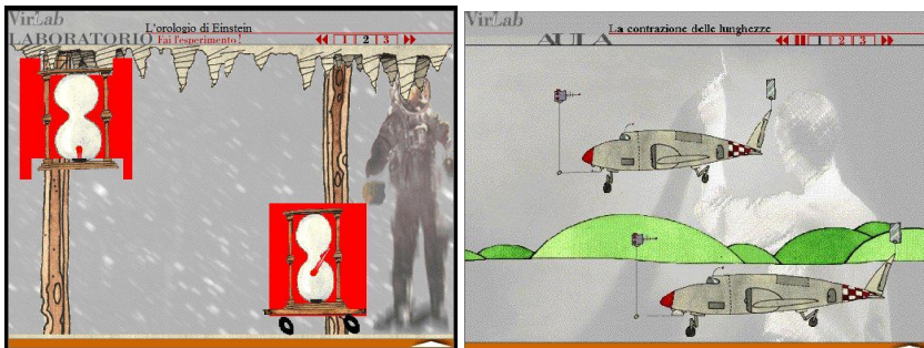
Ryc. 2.5. Zasady szczególnej teorii względności: ciała w ruchu wydają się krótsze, czas na zegarach będących w ruchu zdaje się być spóźniony. Źródło: Ugo Amaldi, „Einstein e la relatività”, CD-Rom, Zanichelli, Padova 1999.
