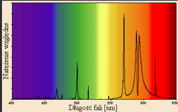
rys. 6 Widmo ulicznej lampy sodowej
