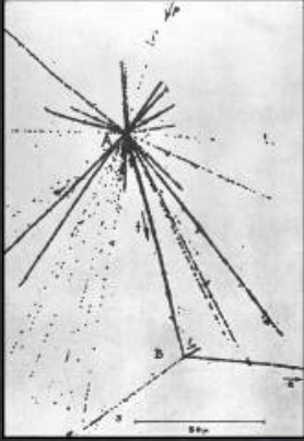
Odkrycie kwarku dziwnego , Danysz i Pniewski, 1956
