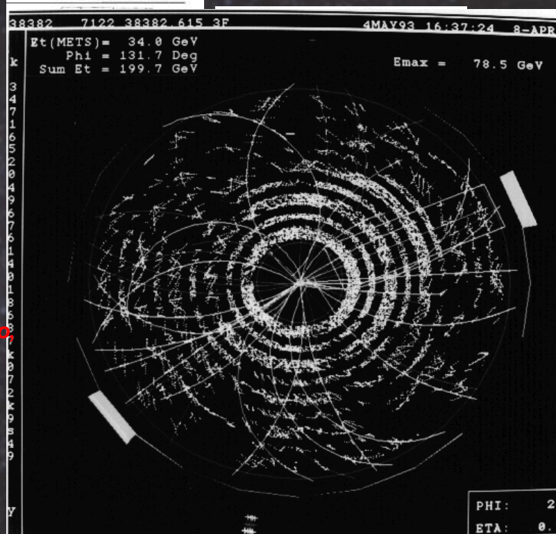
Odkrycie kwarku bottom , FermiLab, Chicago
