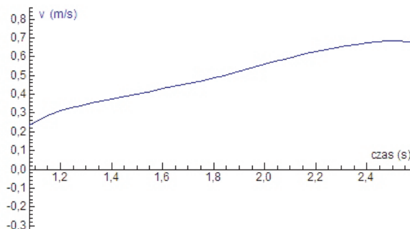
Wykres prędkości wózka w funkcji czasu dla zjeżdżającego wózka.
