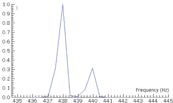
Rys. 5. Widmo częstotliwości badanej fali akustycznej.
