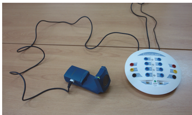
Rys. 1. Sposób podłączenia ultradźwiękowego czujnika położenia do konsoli pomiarowej Coachlab II (foto A. Karbowski).
